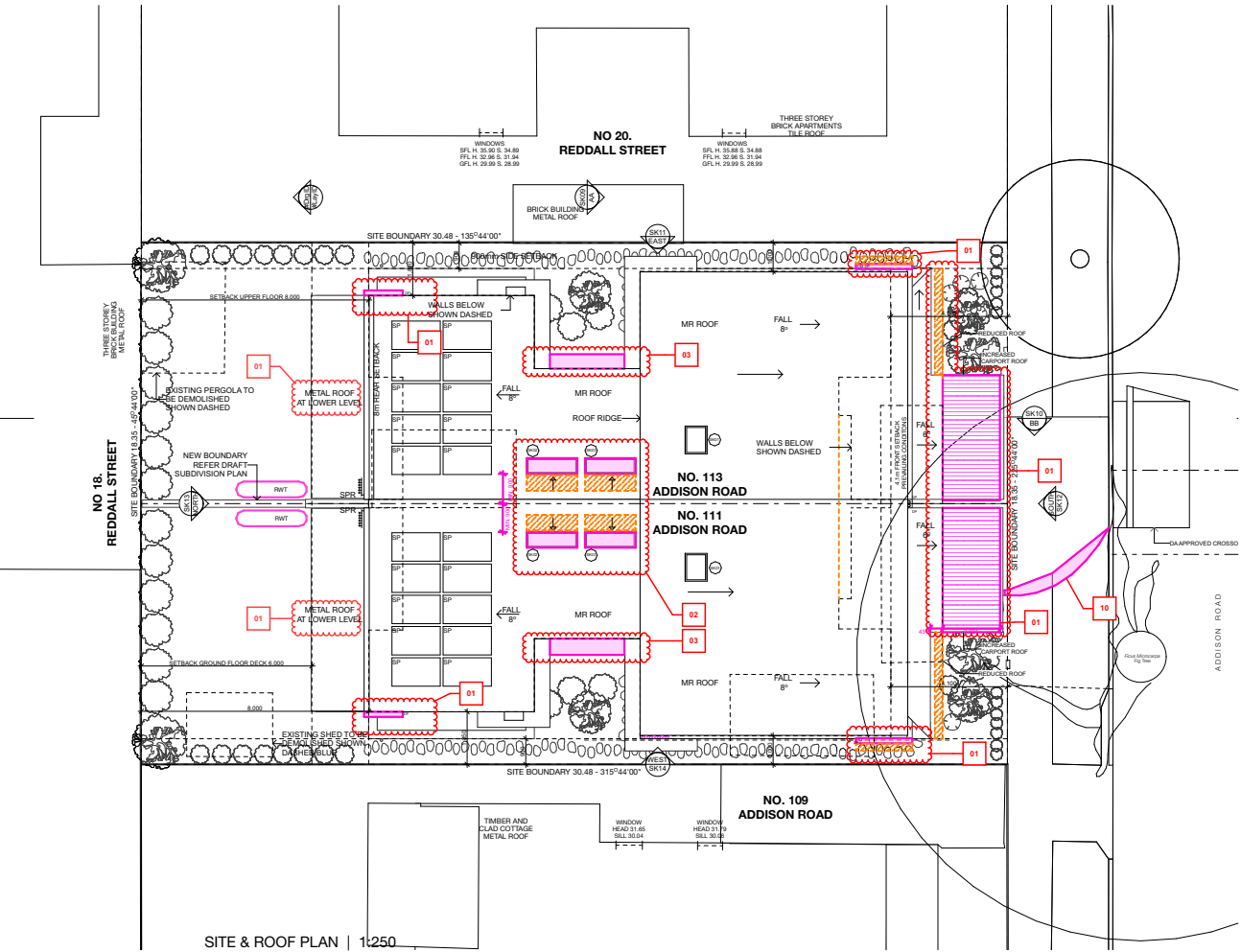
SITE & ROOF PLAN | 1:250
