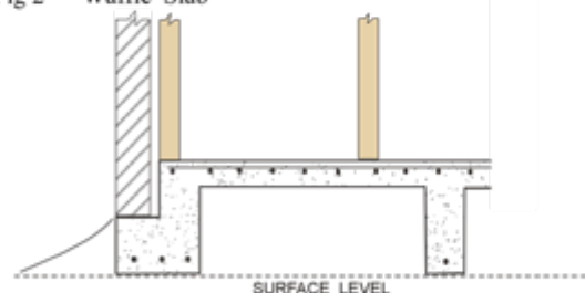
Fig 2 Waffle Slab
