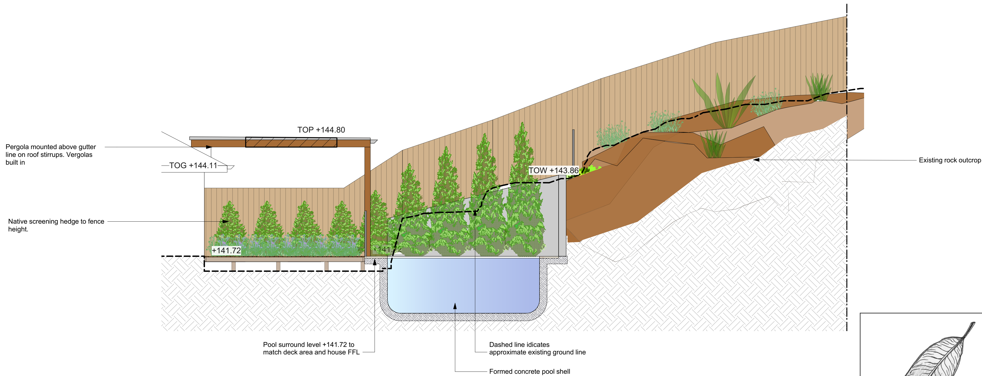
Section DD 1:50@A1 1:100@A3.
