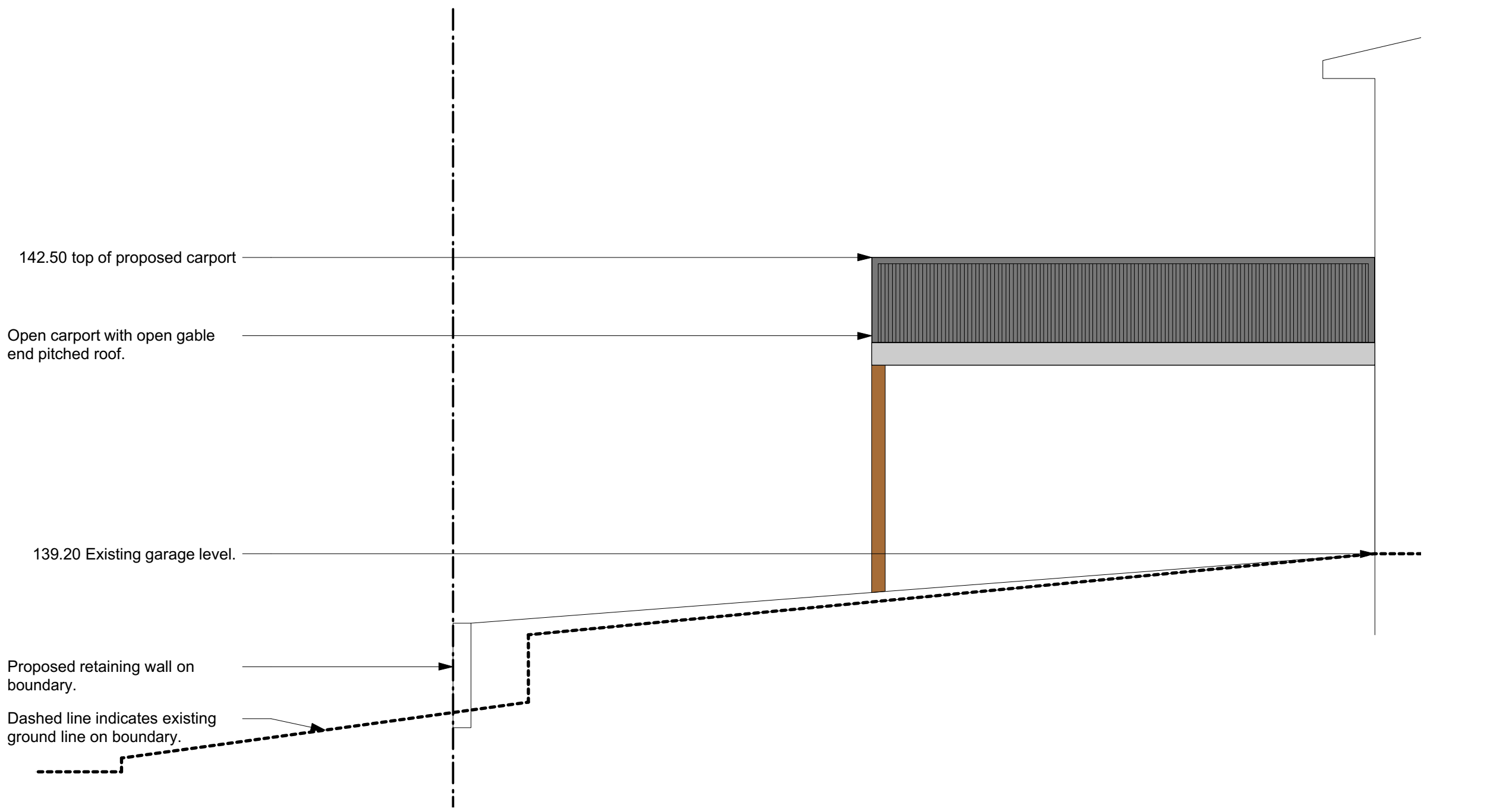
Elevation EE 1:50@A1 1:100@A3.
