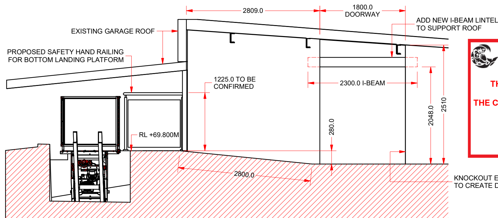
SECTION B-B SCALE 1 : 50
