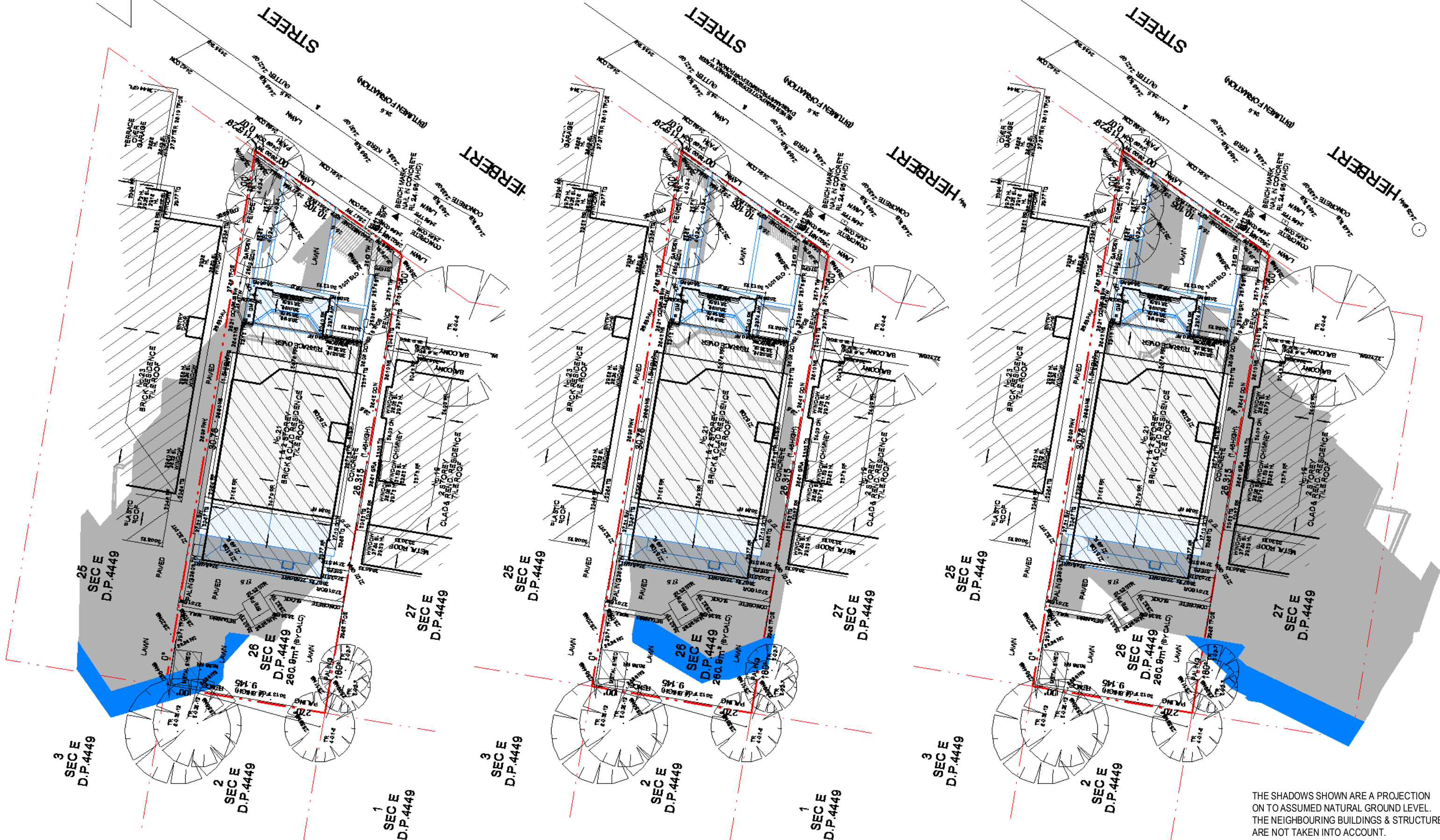
9AM JUNE 21 - SHADOW DIAGRAM 1 : 200
