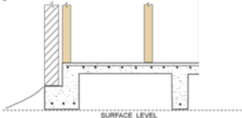
Fig 2 Waffle Slab
