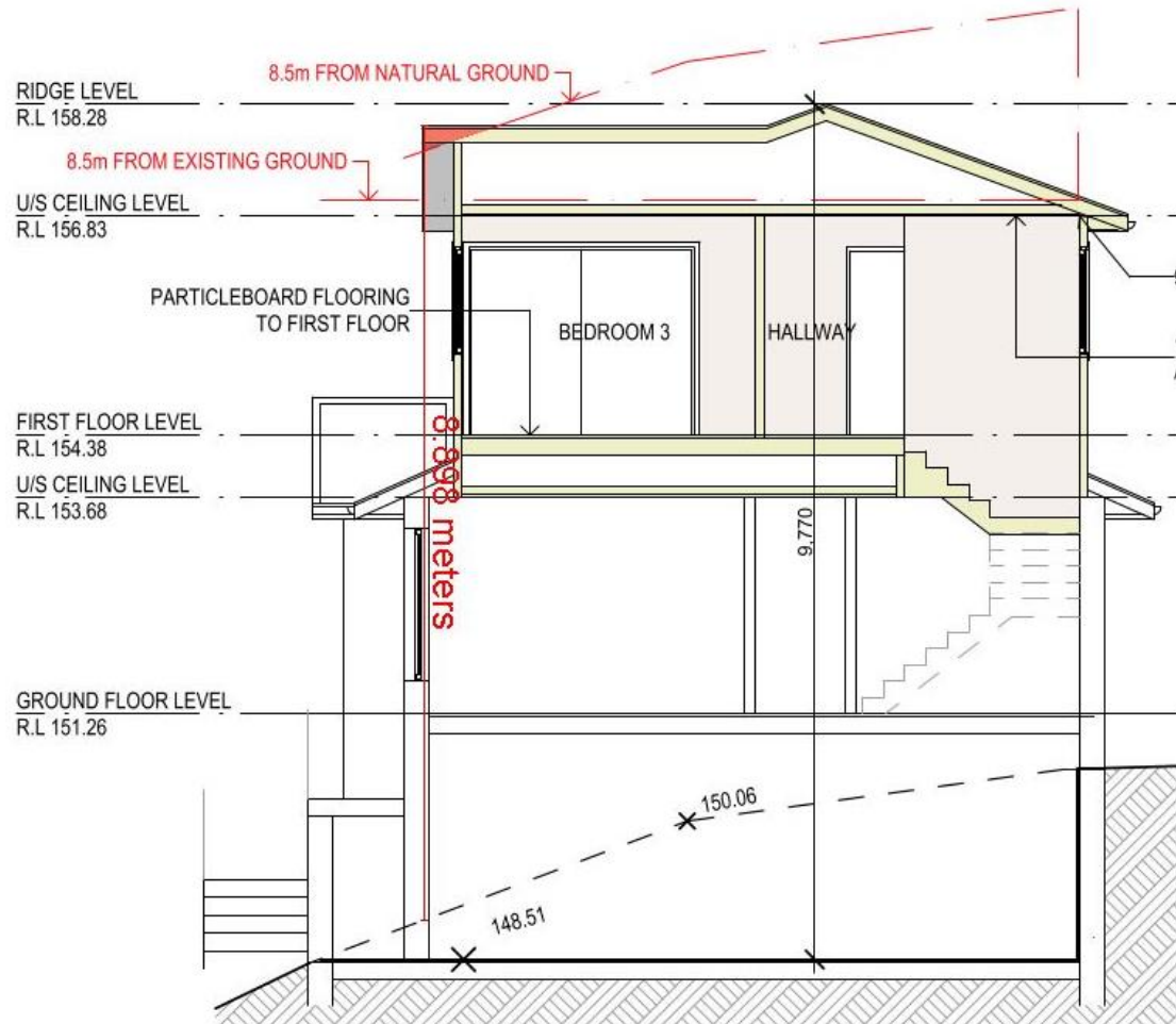
SECTION A-A
