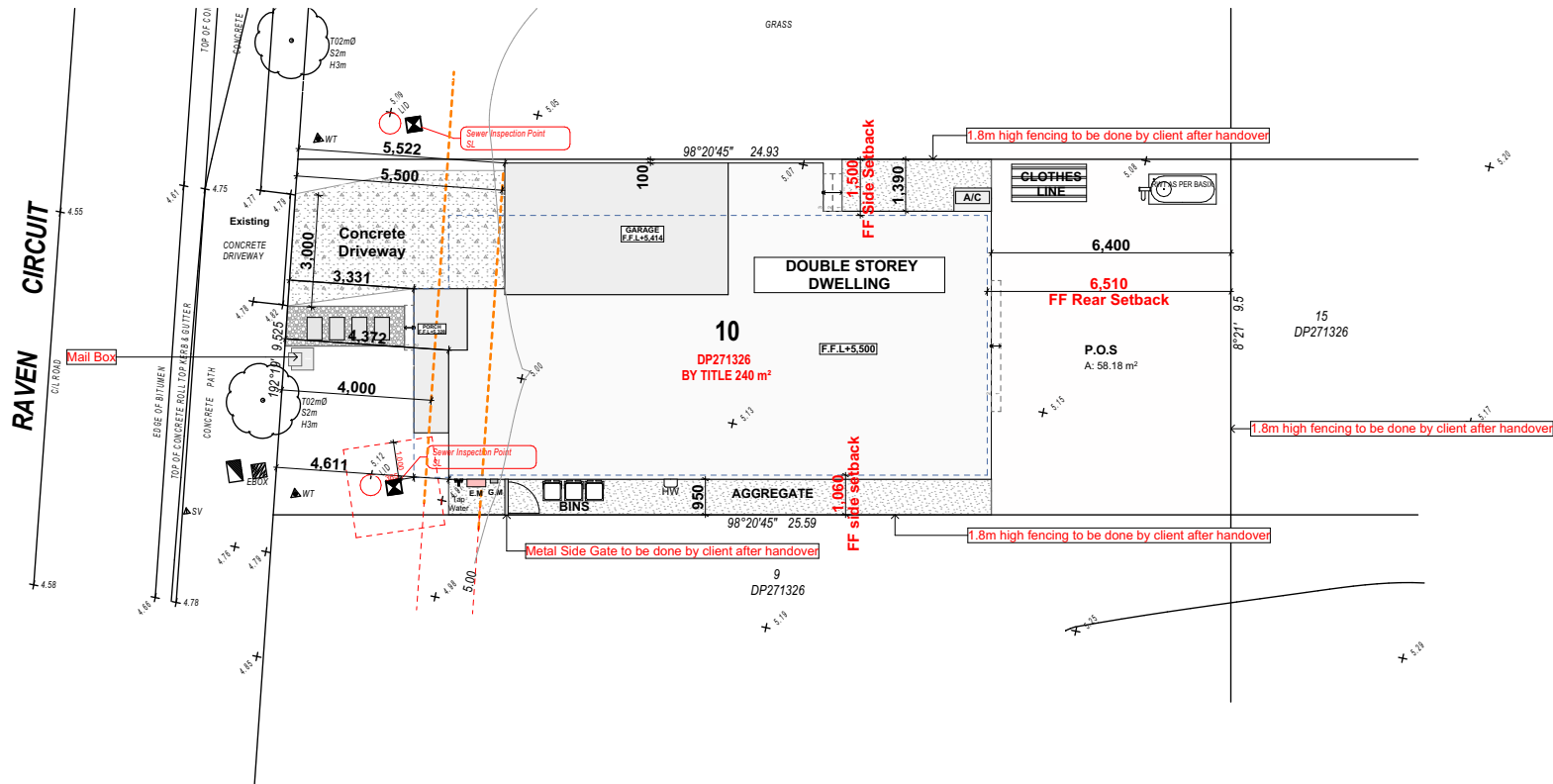
Site Plan 1:200
