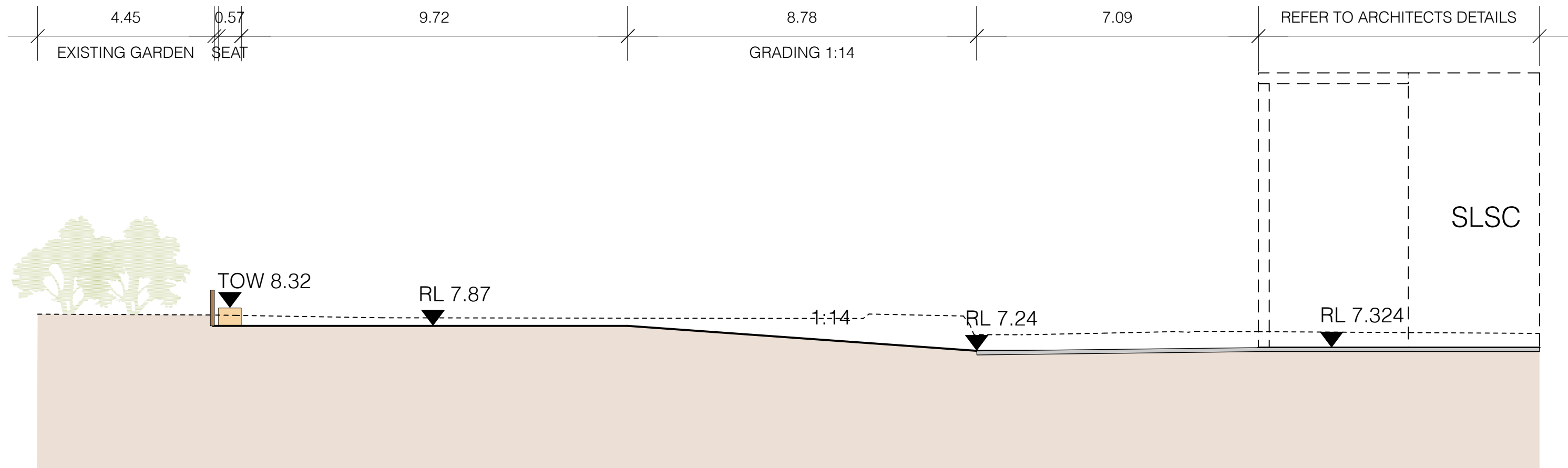
1 SECTION A-A Scale: 1:100
