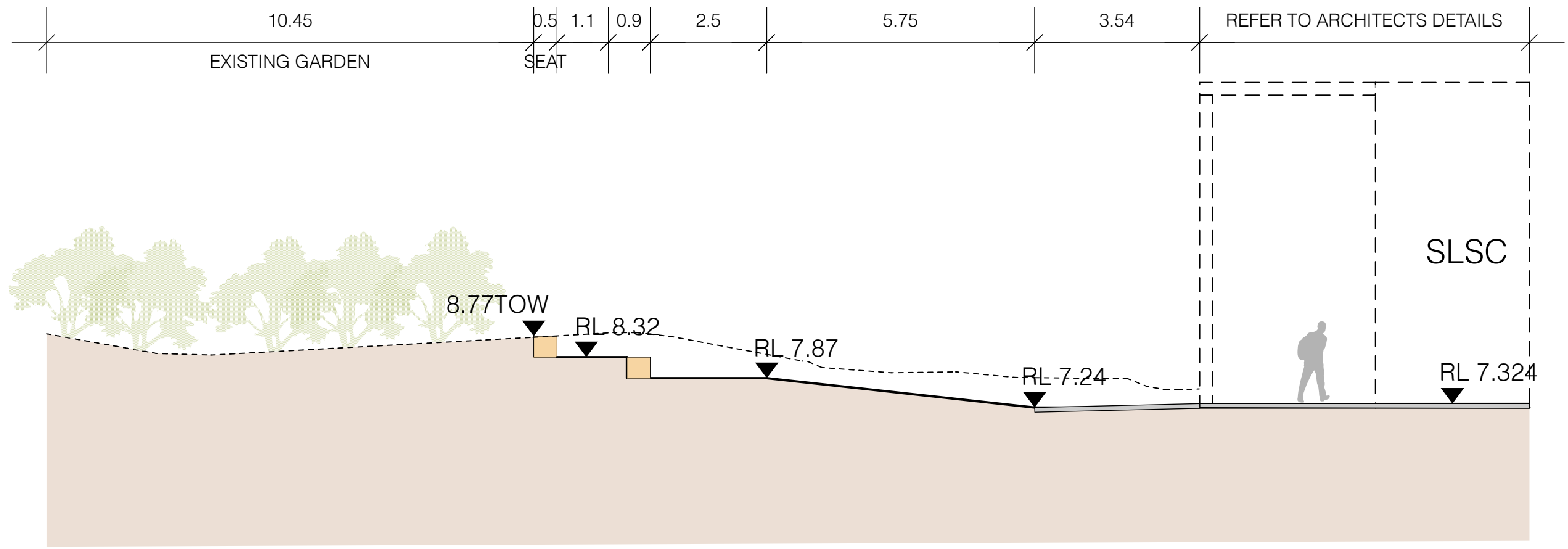
2 SECTION B-B Scale: 1:100
