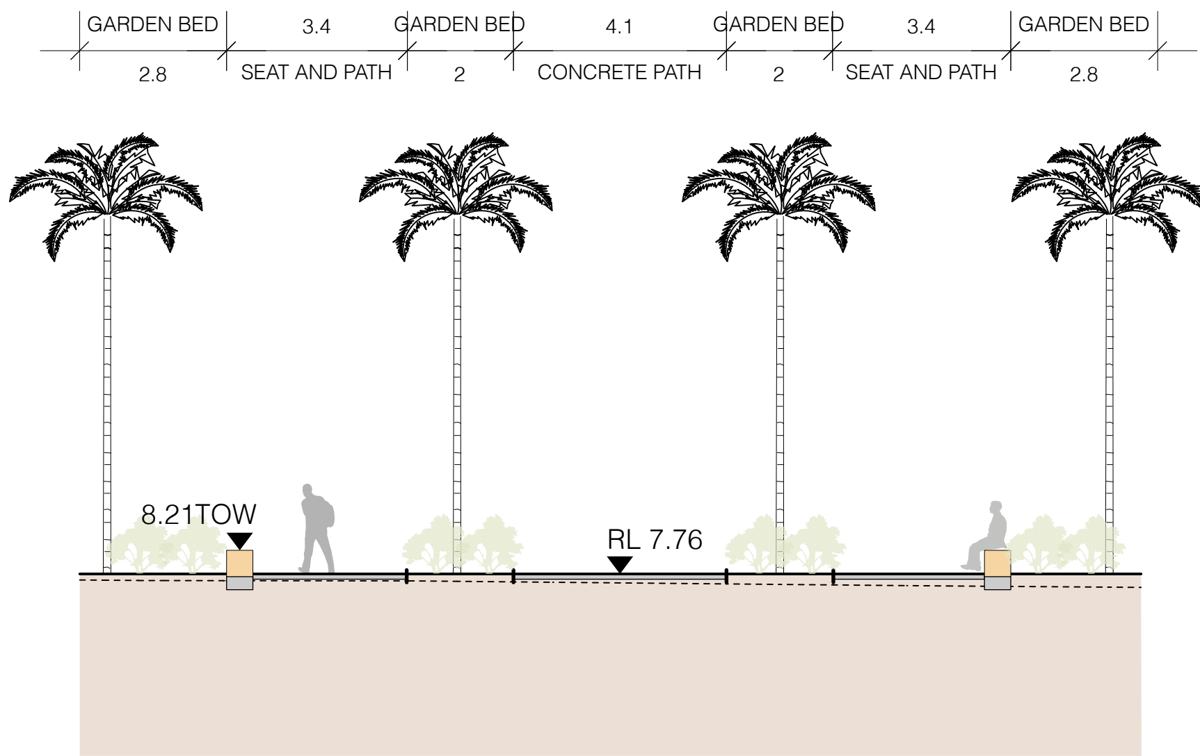
3 SECTION C-C Scale: 1:100
