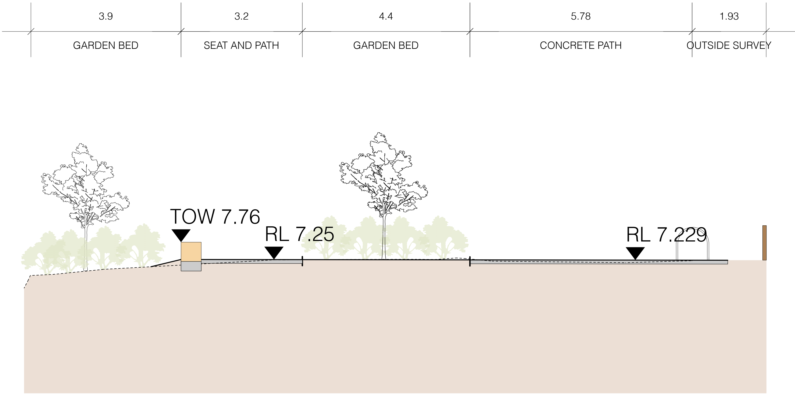
5 SECTION E-E Scale: 1:50
