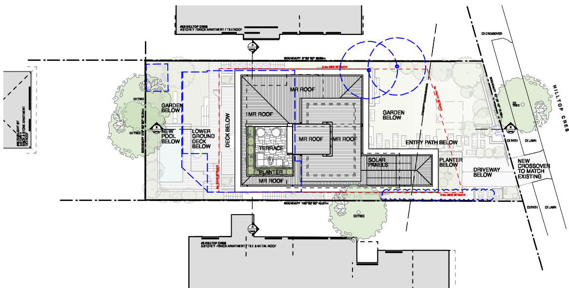
Site Plan 1:400
