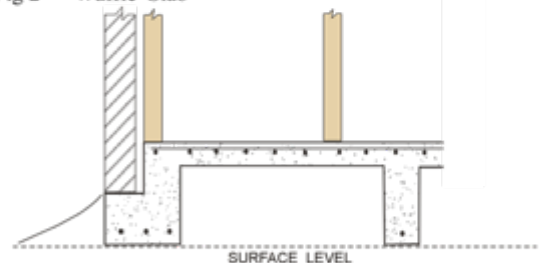
Fig 2 Waffle Slab
