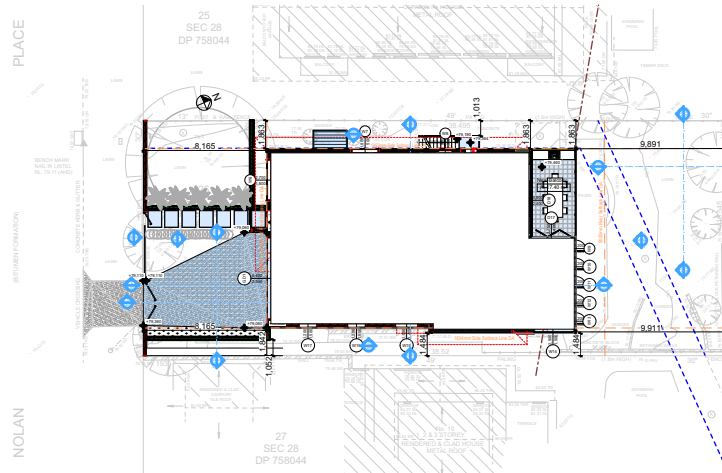
SITE PLAN 1:500
