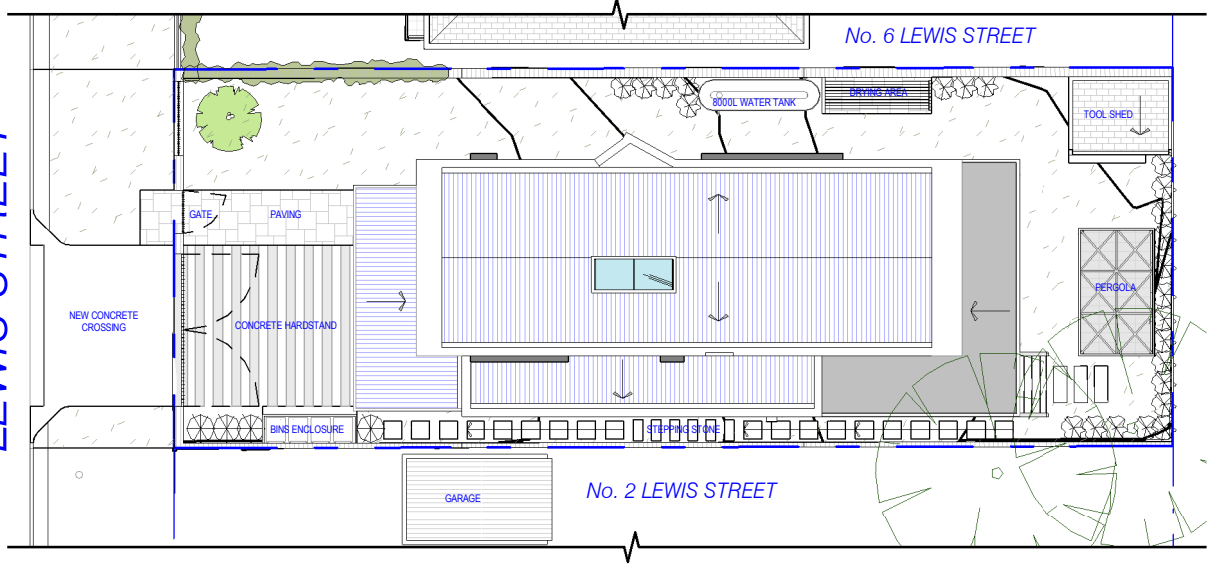
SITE PLAN 1:250
