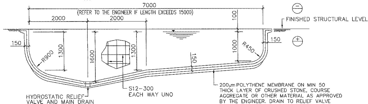
LONGITUDINAL SECTION 1:50
