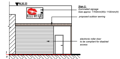
ELEVATION 2 SCALE: 1:200
