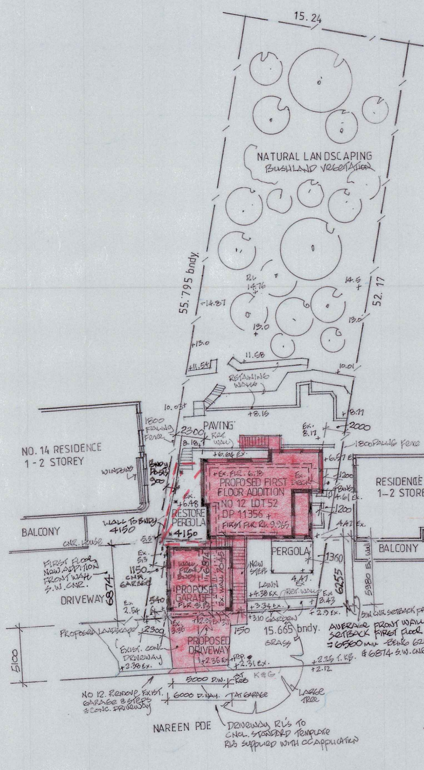
SITE PLAN 1:200
