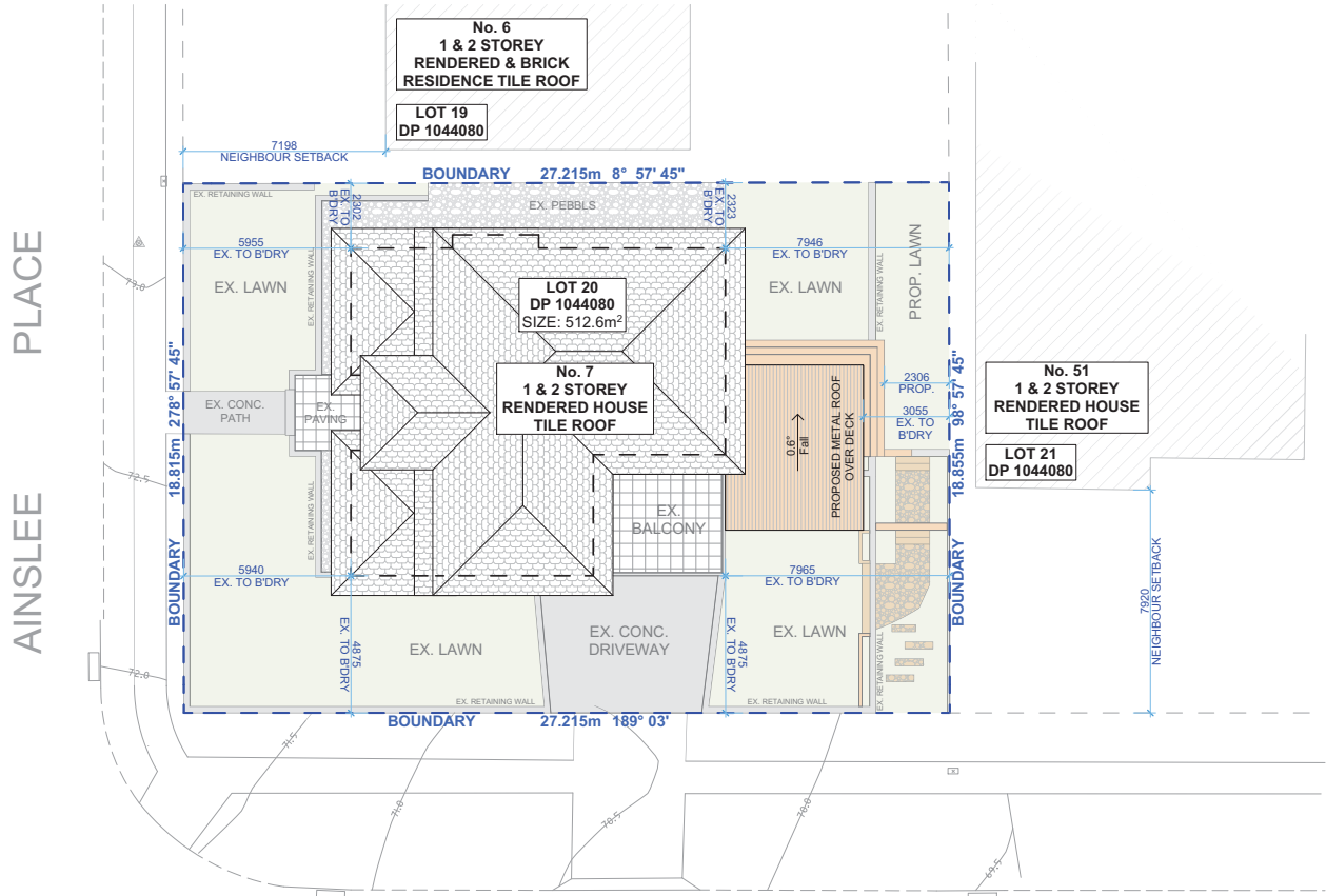
1 SITE PLAN 1:200
