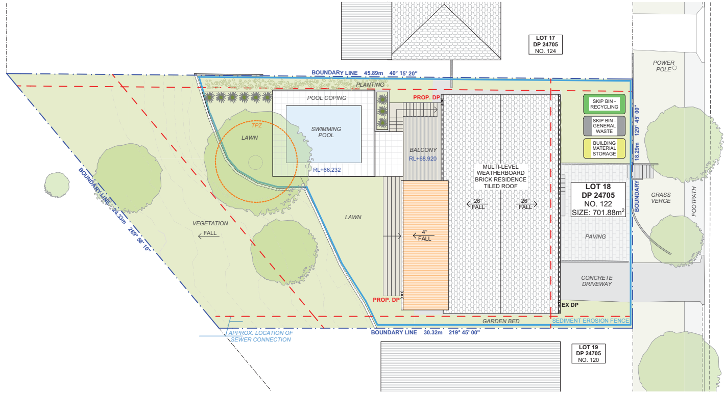
1 SITE PLAN 1:200
