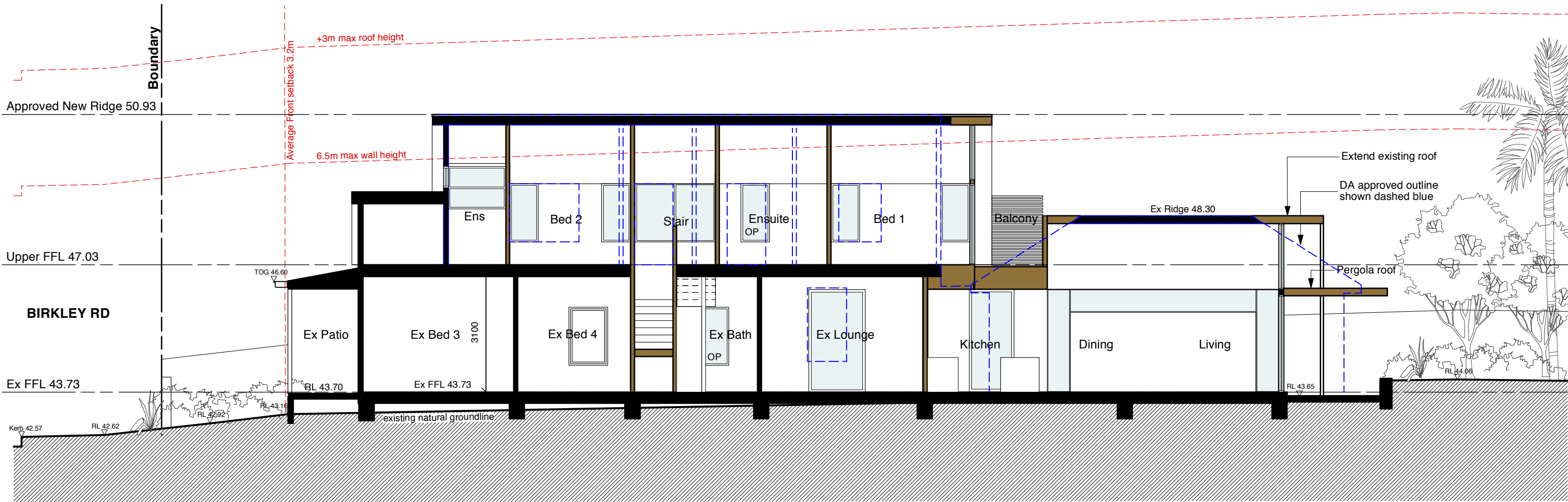
Section A-A
