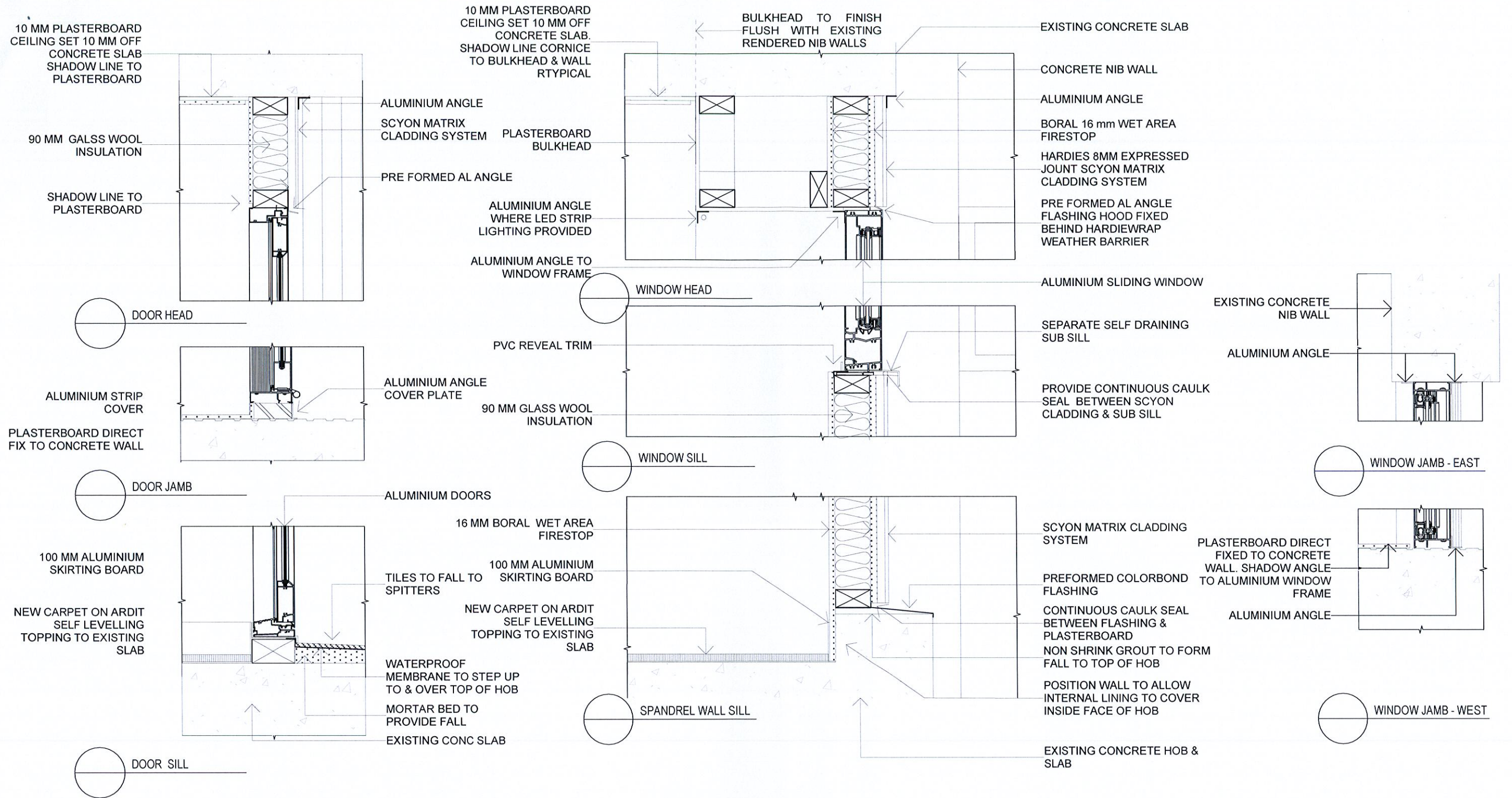
1 DOOR D4 DETAIL WALL TYPE 4 ABOVE DOOR
