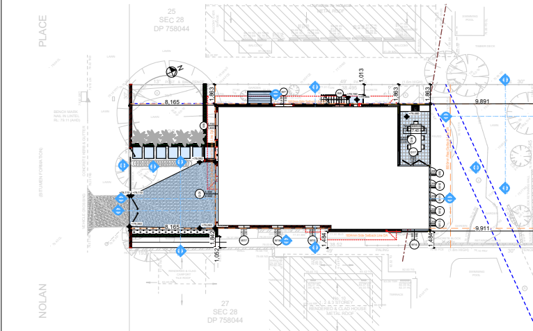
SITE PLAN 1:500
