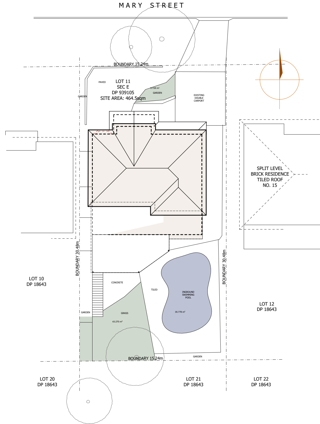
SITE PLAN 1:200
