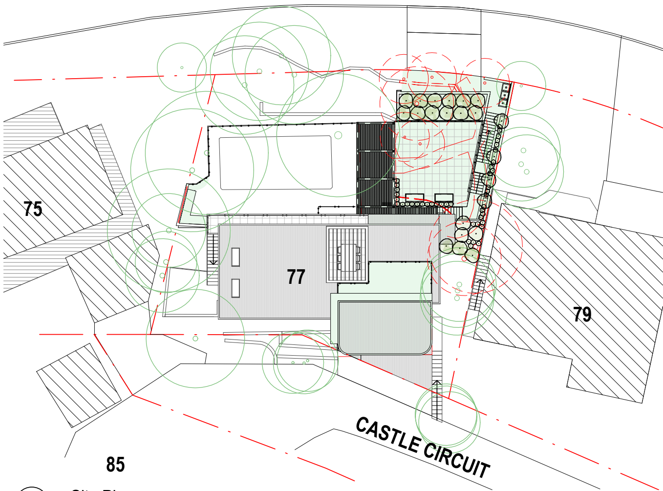
1 Site Plan 1 : 300
