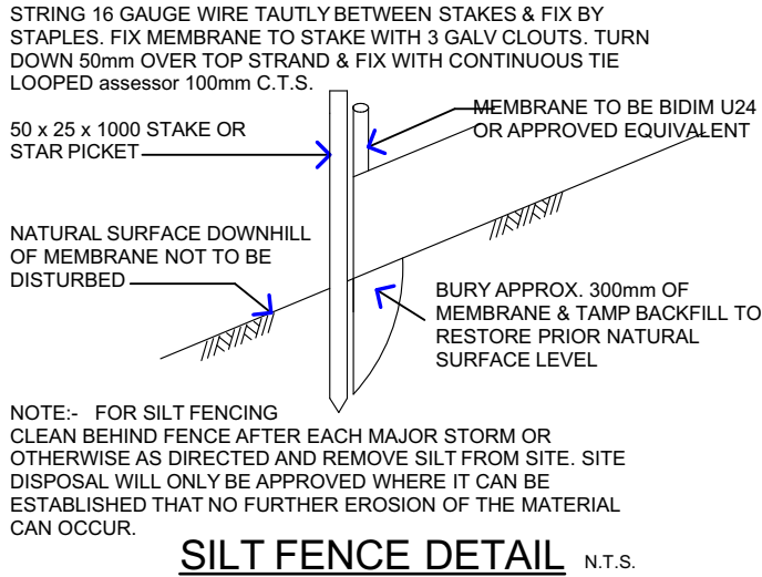
SILT FENCE DETAIL N.T.S.
