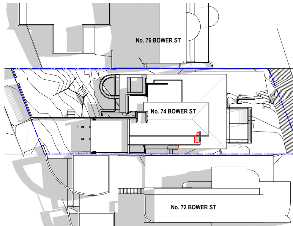
5 WINTER 1200 Scale: 1:400
