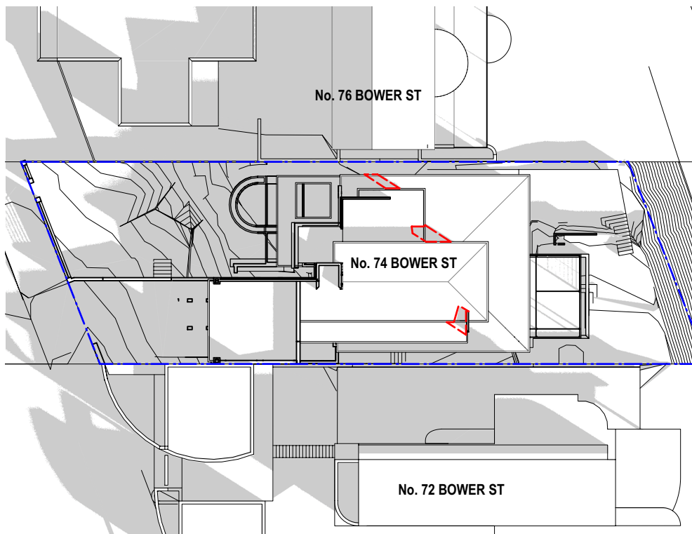
4 WINTER 0900 Scale: 1:400
