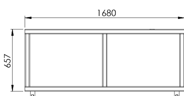
TOP HEADER FRAME QTY: 1
