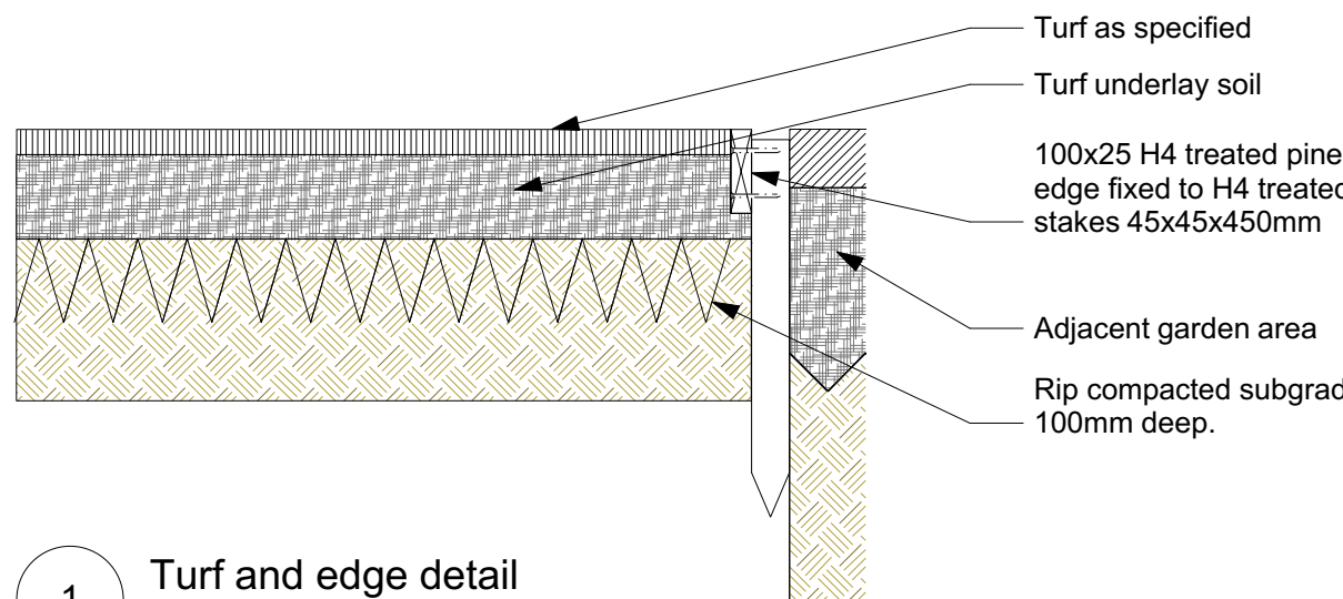
1 Turf and edge detail Scale: 1:10
