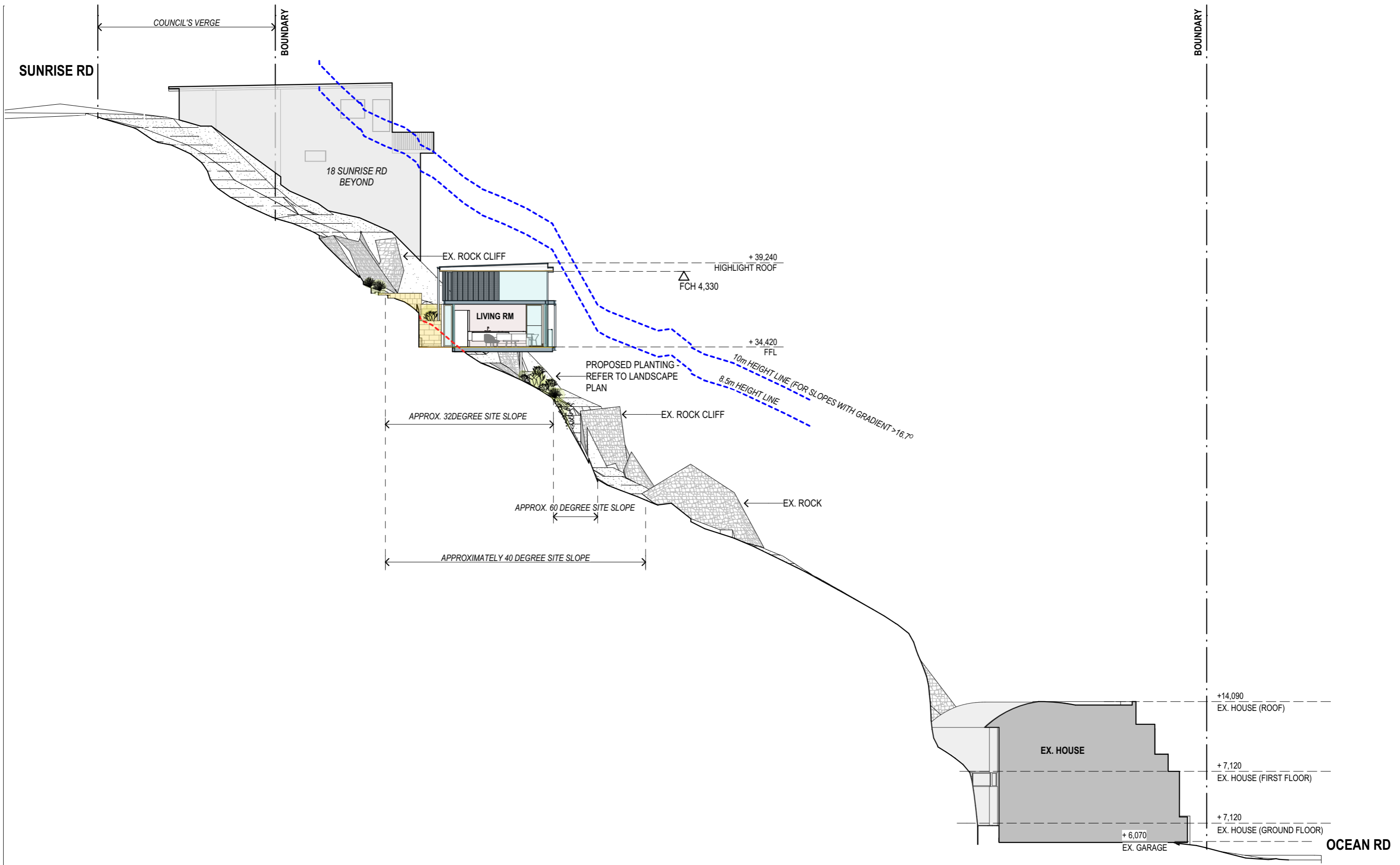
1 SITE SECTION 1:200
