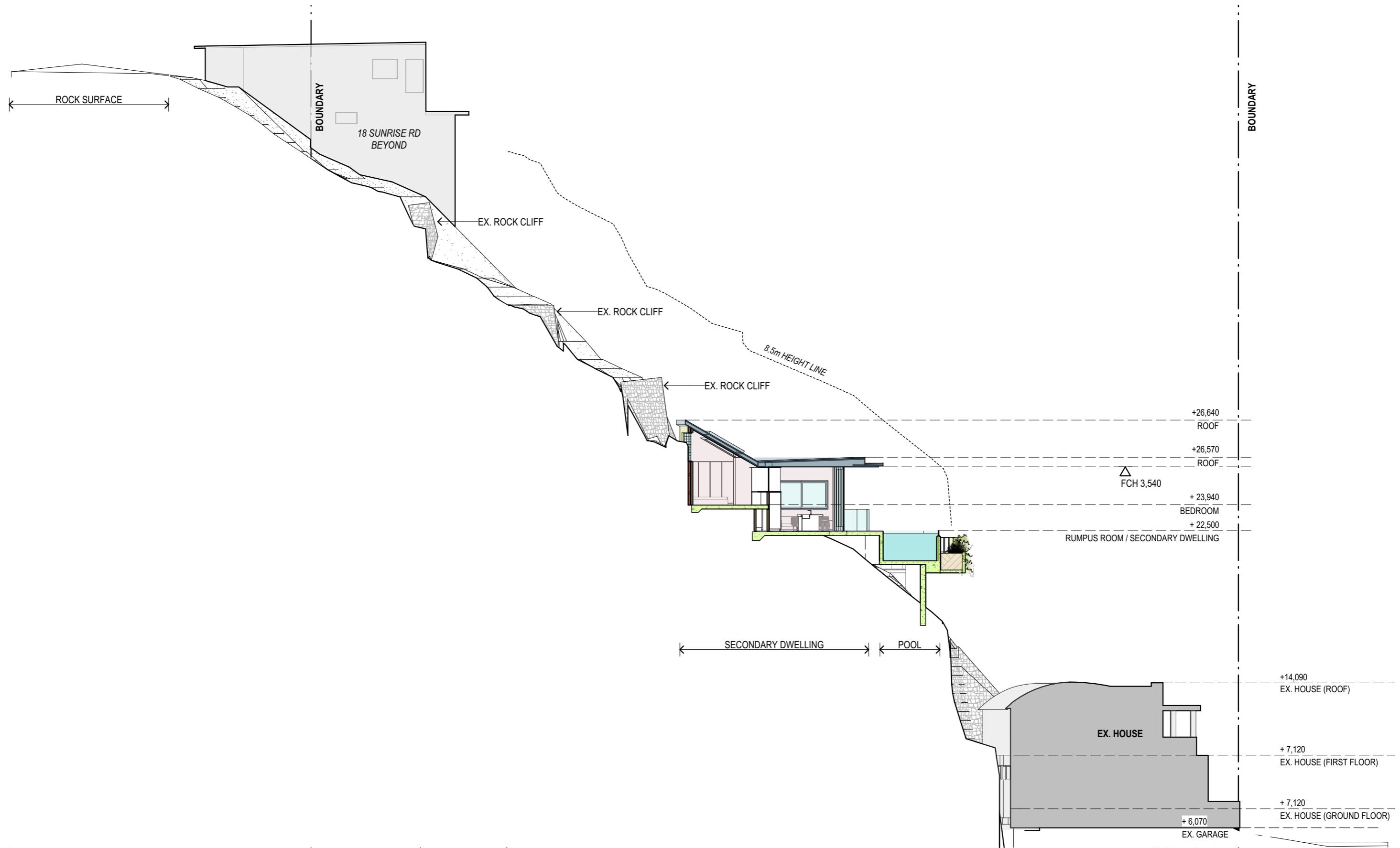
1 SITE SECTION 1:200
