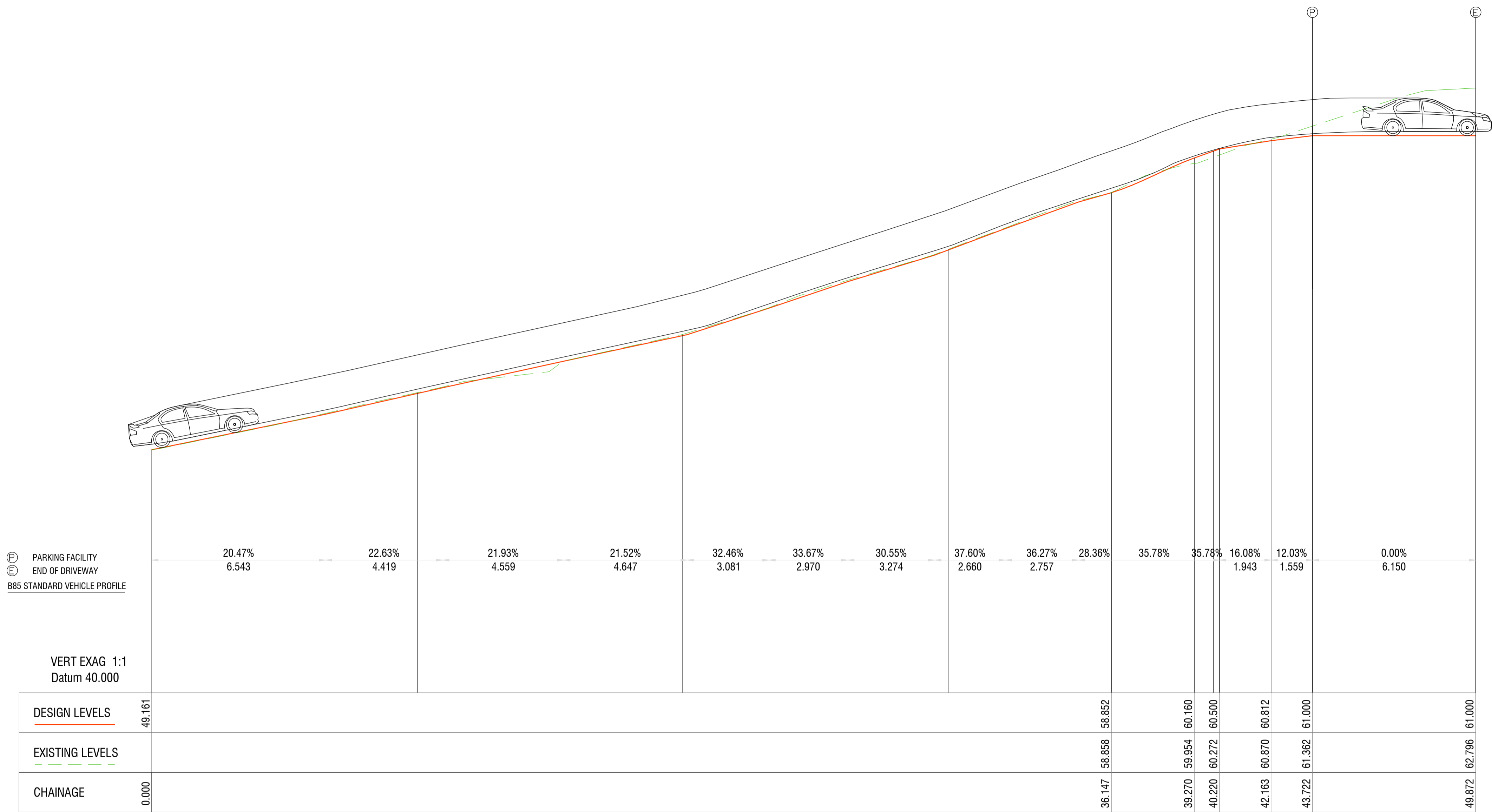
LEFT EDGE LONG SECTION
