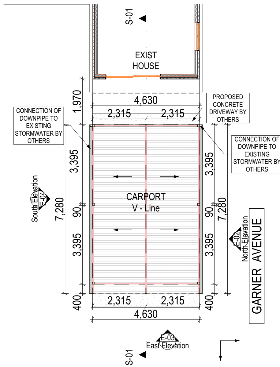
Carport Plan 1:100
