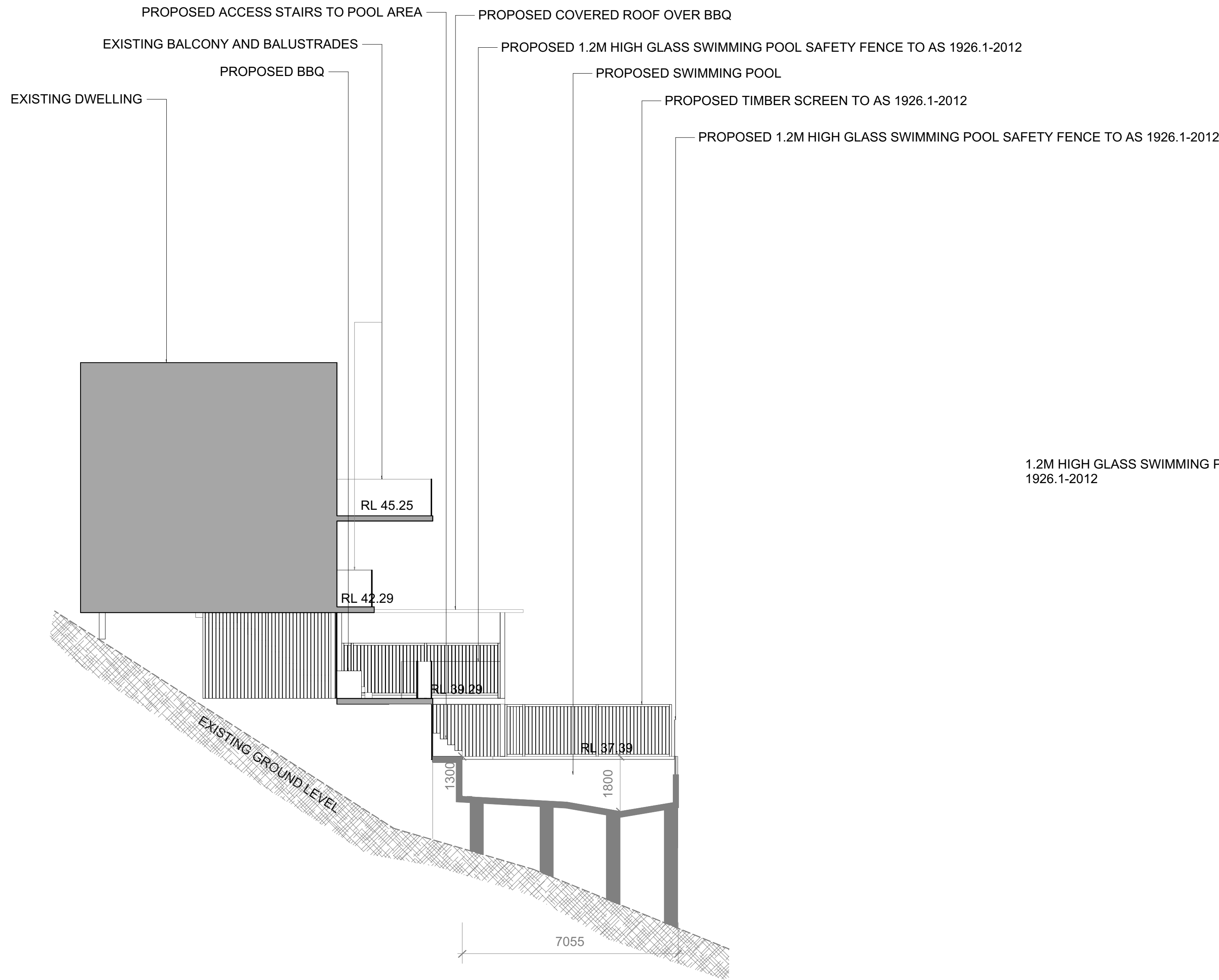
1 SECTION AA Scale: 1:100
