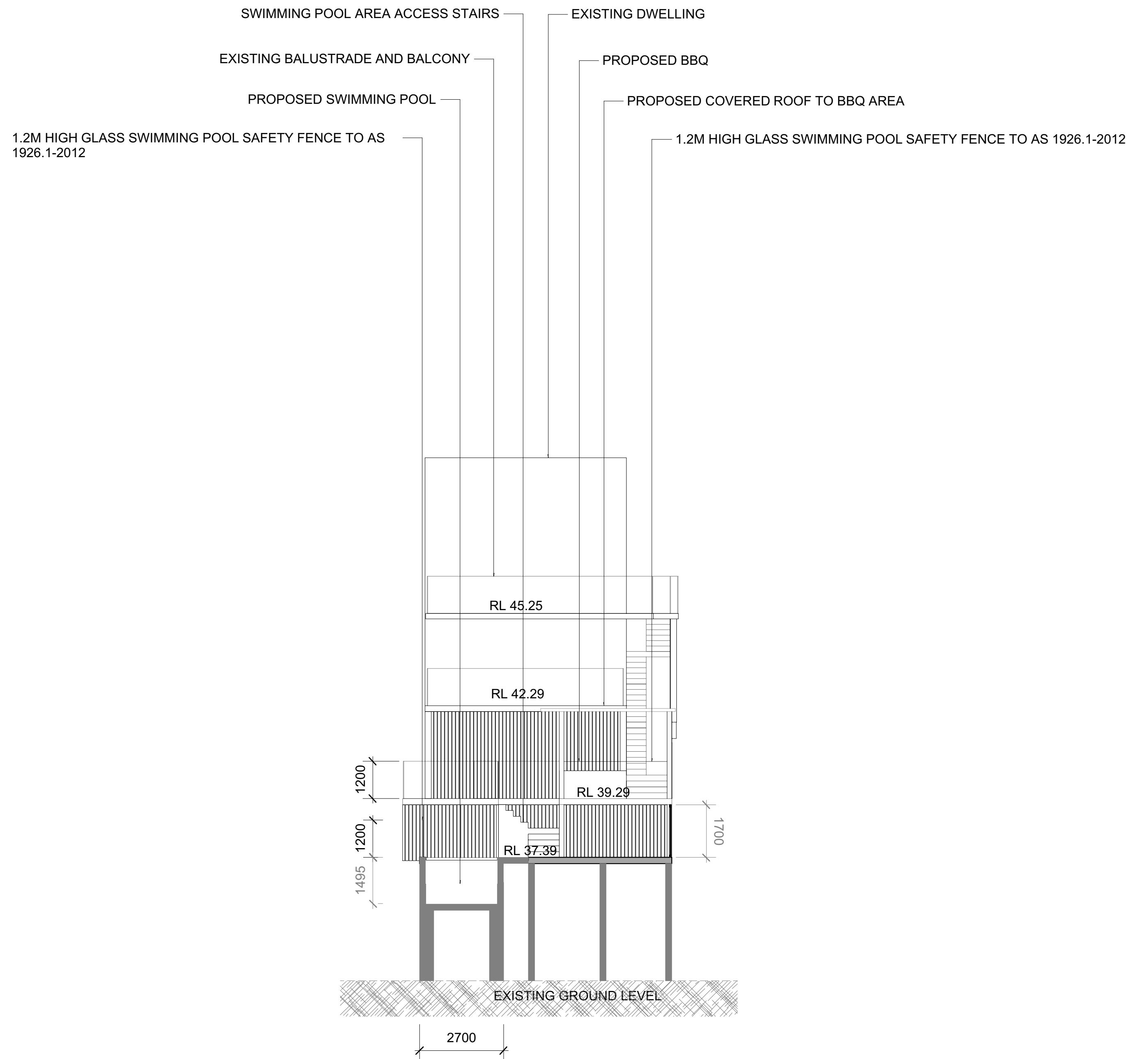
2 SECTION BB Scale: 1:100
