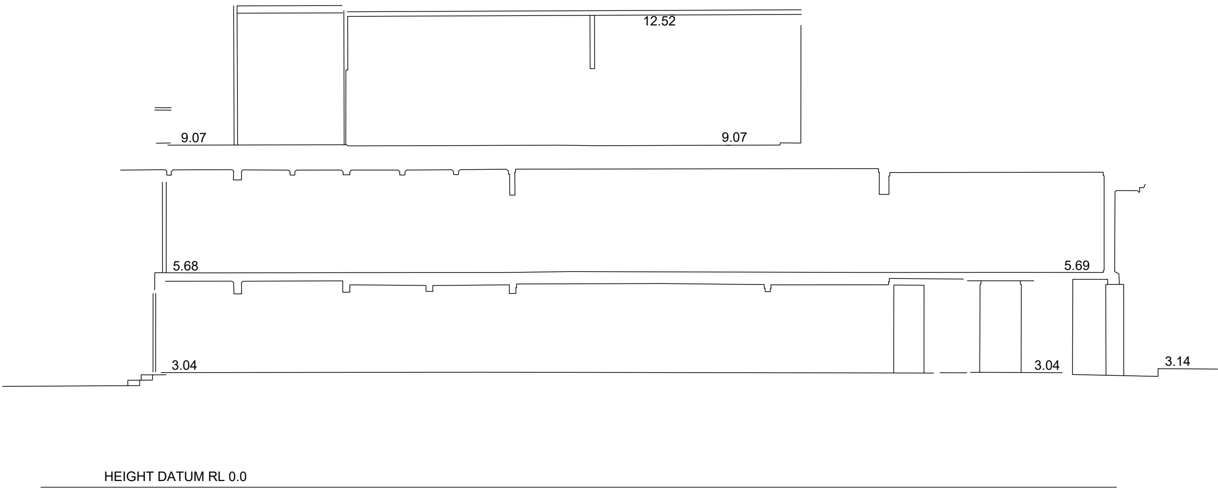
SECTION A-A
