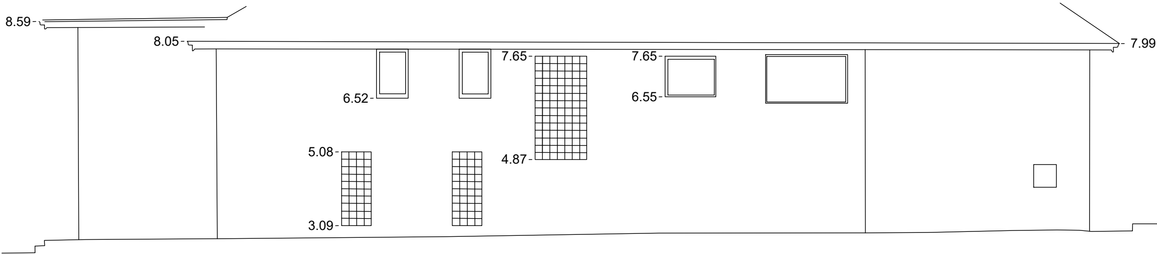
ELEVATION 3
