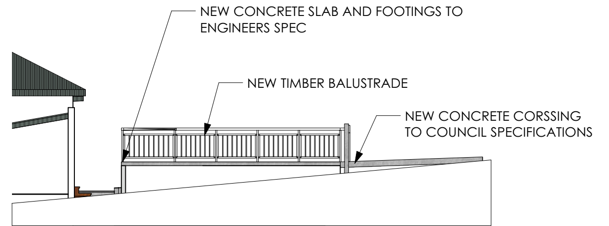
2 WEST ELEVATION Scale: 1:100
