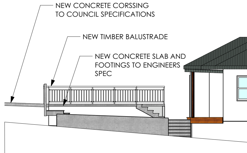
3 EAST ELEVATION Scale: 1:100
