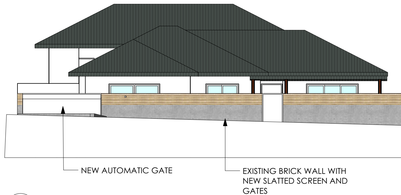
1 SOUTH ELEVATION Scale: 1:100
