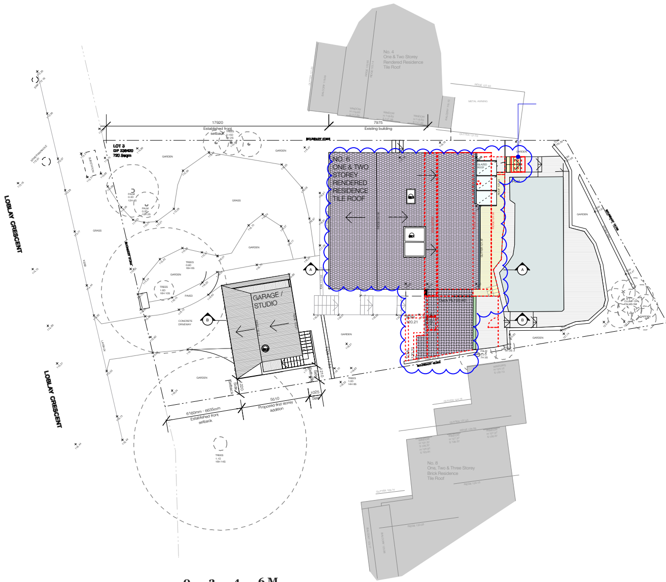
1 Site Plan NTS
