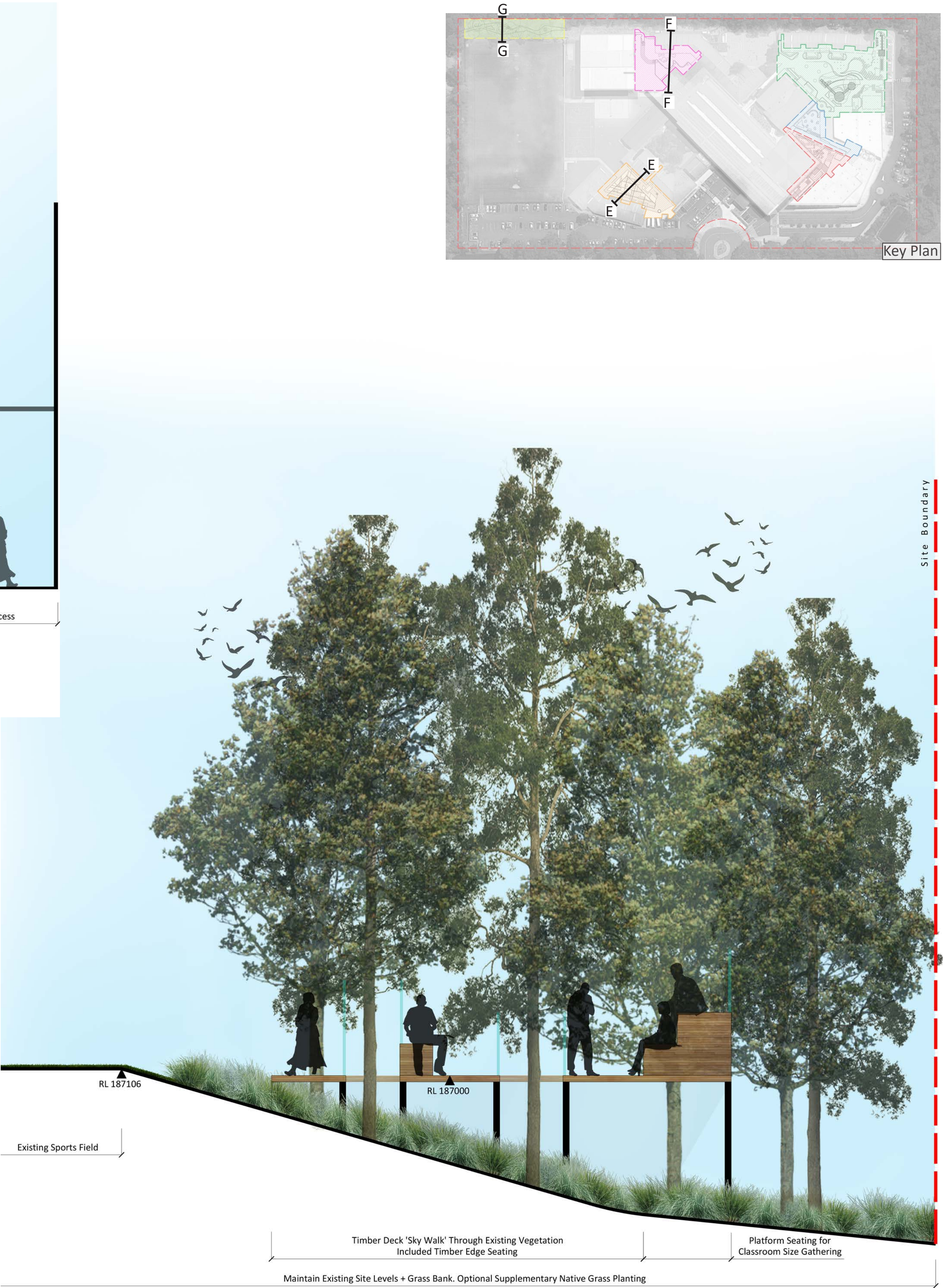
Section GG // Tree Walk // Scale 1:40
