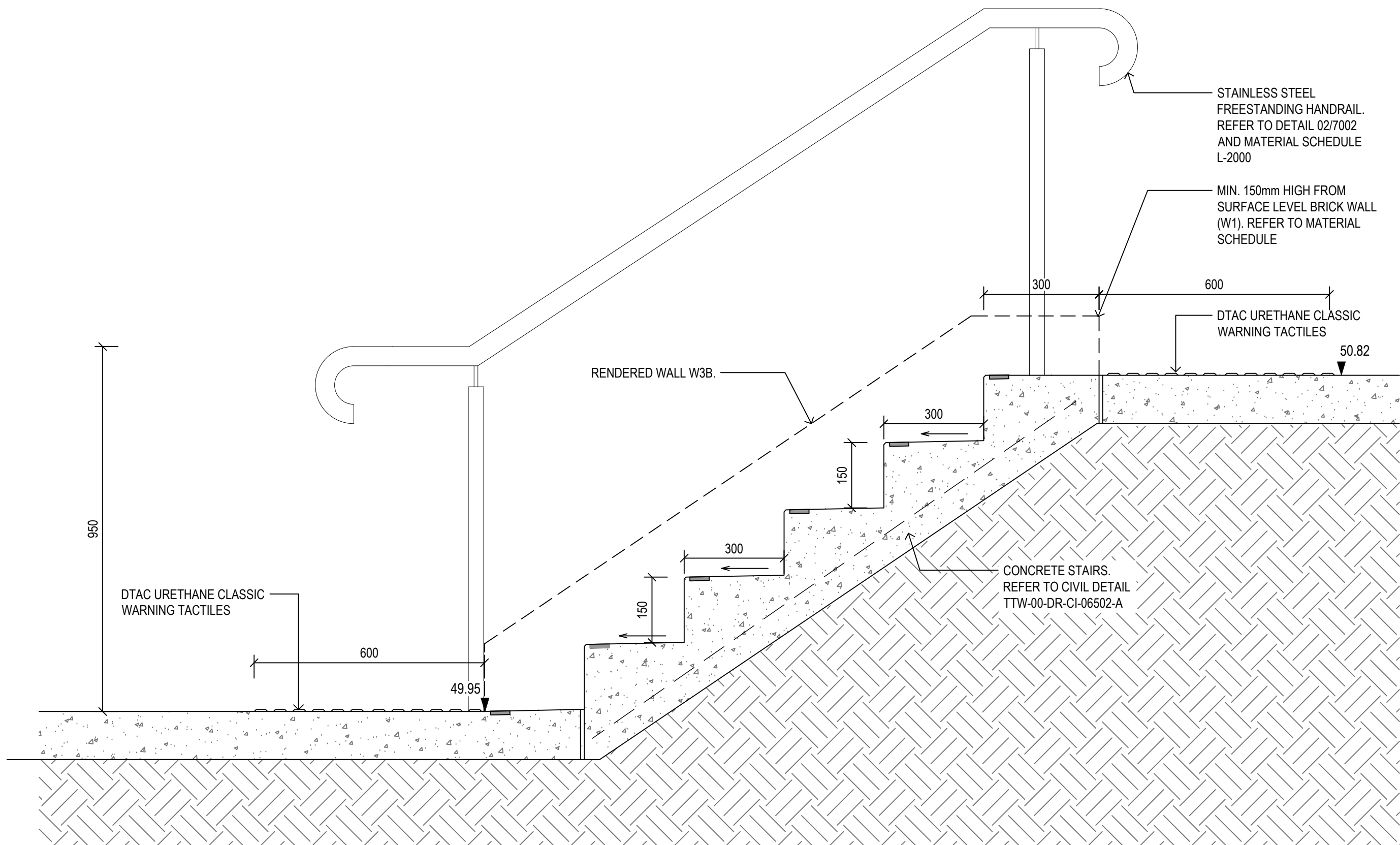
02 STAIR 2 6002 1:10
