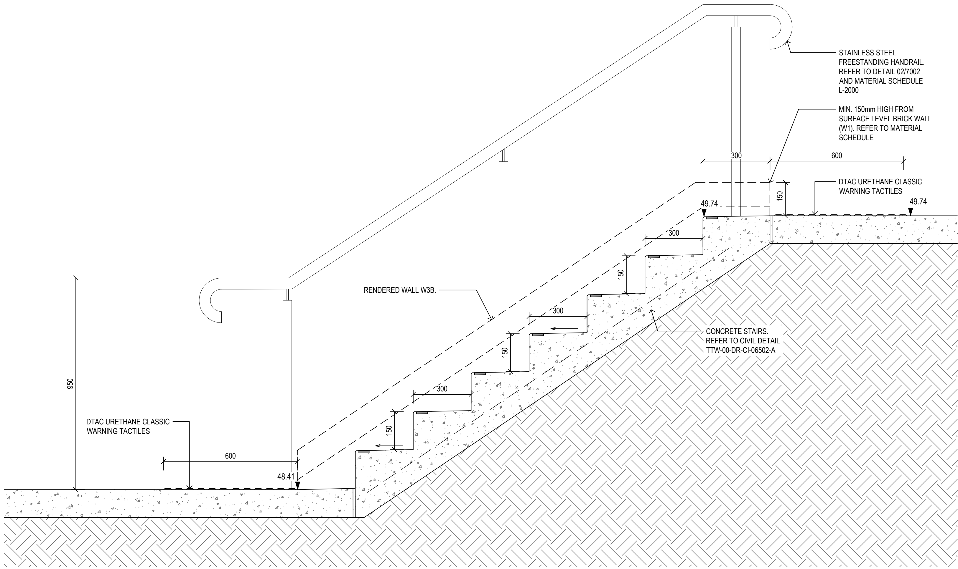
01 STAIR 1 6002 1:10
