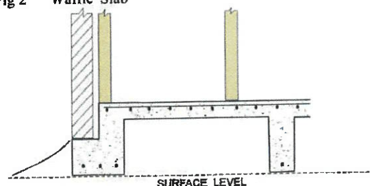
Fig 2 Waffle Slab
