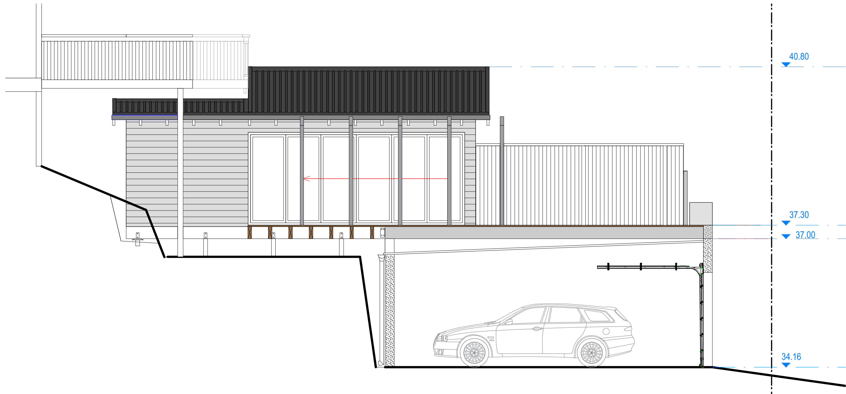
Long Section 1:50@A1 1:100@A3.
